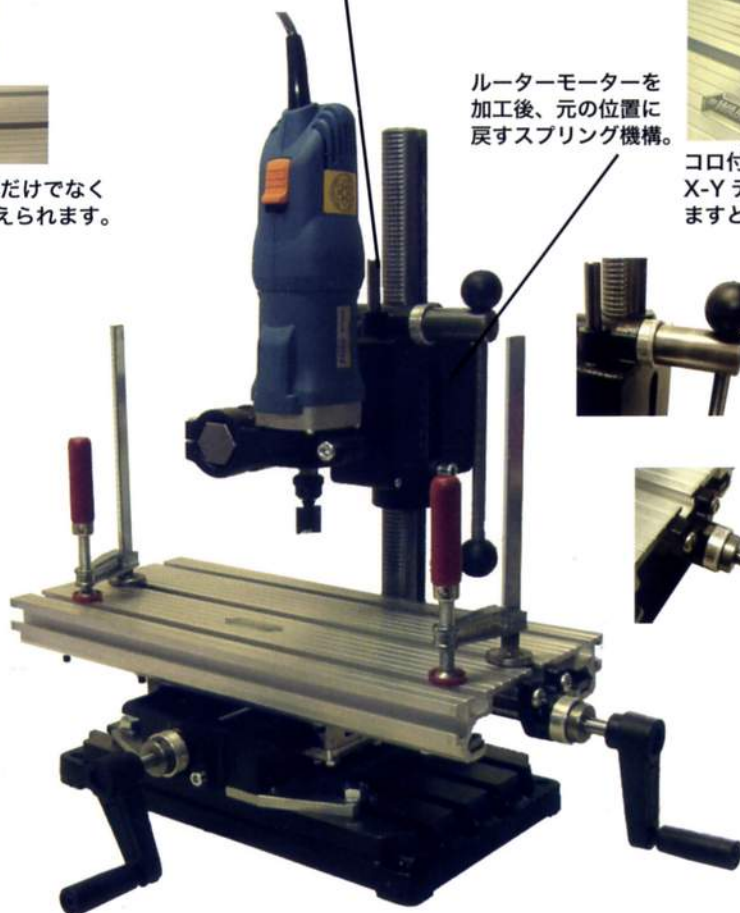
ルーターモーターを上下前後に移動させるハンドルの付け根には移動量わかる1mm単位スケールが付いています。
