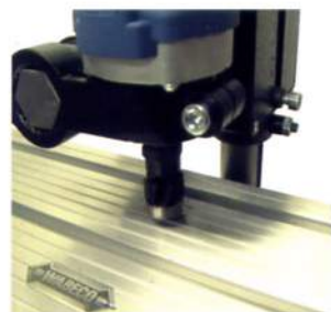
コロ付きルータービットを取り付けてX-Yテーブル上で曲面状の材料を動かしますと、飾り面取り加工ができます。
