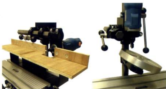
更に別売の木製ミリングテーブル(No. 24430)を右写真のように取り付けますと材料をスライドさせながらの面取り加工ができます。また、ルーターモーターを上下させることでアリ・あられ組み加工も可能です。
