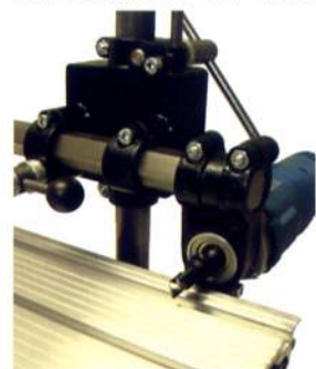
縦コラムを回し、ルーターモーターを水平にすることにより、材料の側面の加工もできます。
