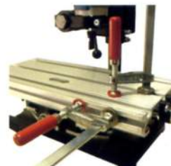
材料を固定する専用バイスはX-Yテーブル上のどここの位置でも固定でき、テーブル側面にも留められます。
