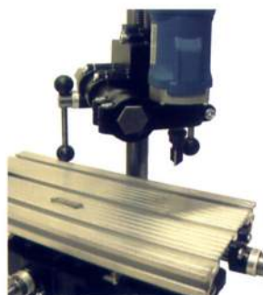
縦コラムの根元のボルトを緩めると角度変えることができるうえ、横コラムを左側のハンドルを使って斜め前後にスライドできます。
