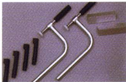
アクセサリーキット (ST03、バイスピ (4)、 アルミ製バイスカバー(2)) 品番 33619
