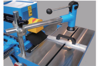
モーター部を前後左右に動かすハンドルには等間隔ドリルガイドピンを操作できるレバーが付いているので、スピーディに多数のダボ穴があげられます。
